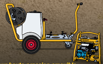
Nettoyeur haute pression amovible Le chassis porteur du nettoyeur haute pression se détache aisément pour faciliter l'entretien et le transport.
